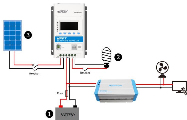
Kuva 2-2 Kytentäkaavion malli
