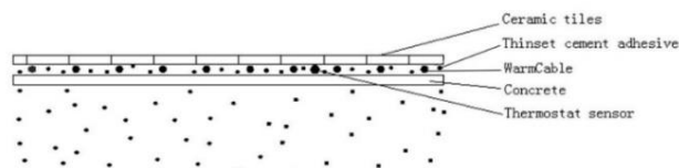
Kuva 2: Suoraan betoniin
