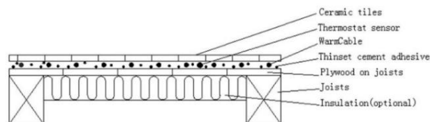
Kuva 1: Suoraan vaneriin
