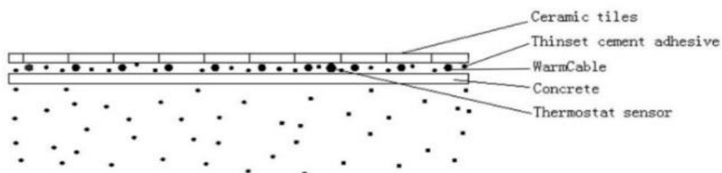
Kuva 2: Suoraan betoniin
