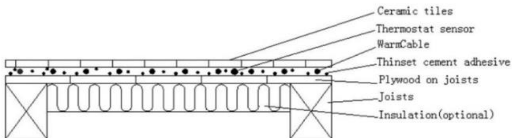
Kuva 1: Suoraan vaneriin
