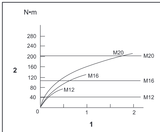
1. Åtdragningsmoment 2. Åtdragningsmoment
