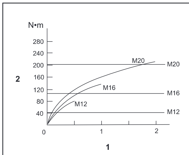
1. Åtdragningsmoment 2. Åtdragningsmoment
