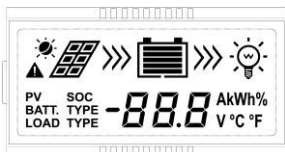
Kuva 3-1 LCD-näyttö
