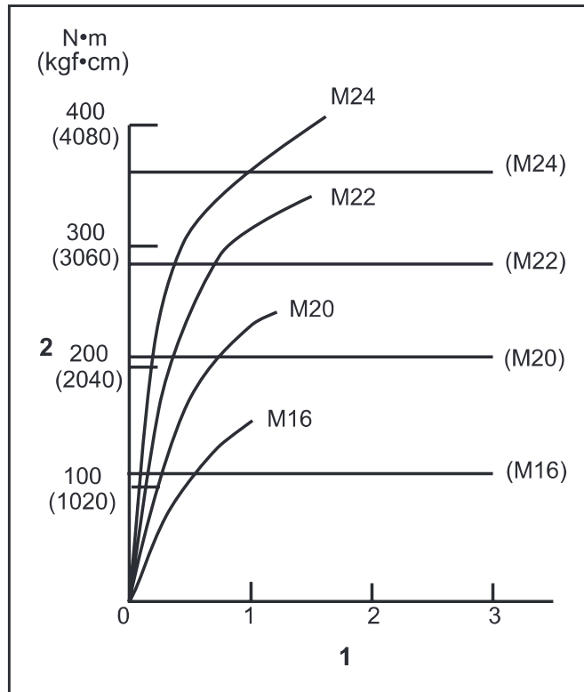
1. Åtdragningsstid (sekunder) 2. Åtdragningsmoment
