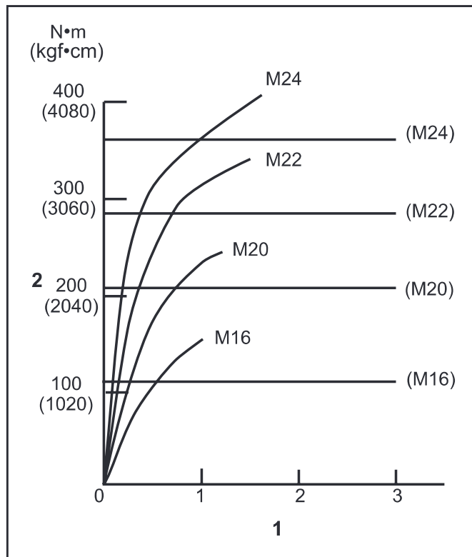
1. Kinnitamisaeg (sekund) 2. Väändemoment
