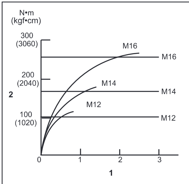
1. Kiinnitysaika (sekunneissa) 2. Kiinnitysvääntömomentti
