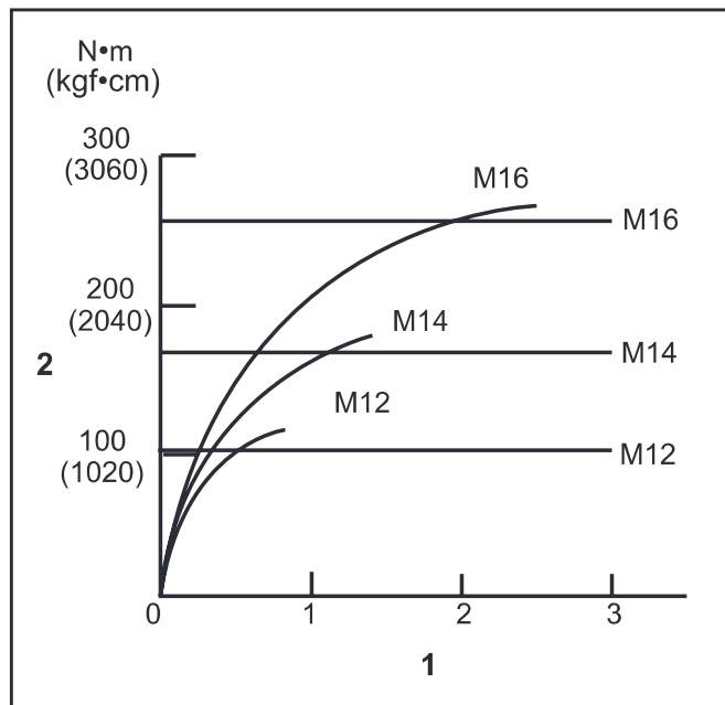
1. Åtdragningsstid (sekunder) 2. Åtdragningsmoment
