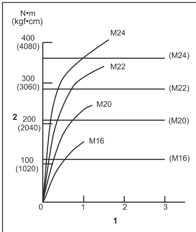
1. Время затяжки (с) 2. Момент затяжки
