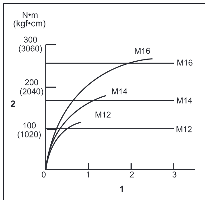
1. Pievilkšanas laiks (sekundēs) 2. Pievilkšanas griezes moments
