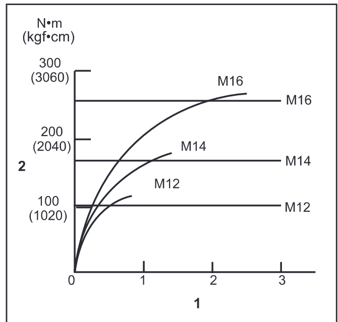
1. Užveržimo laikas (sekundėmis) 2. Užveržimo sukimo momentas
