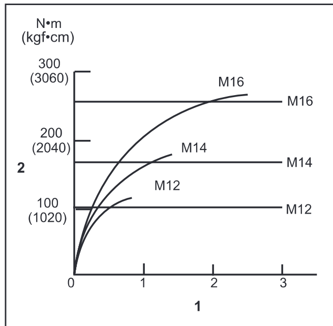
1. Время затяжки (с) 2. Момент затяжки
