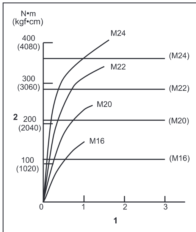
1. Tilspændingstid (sekunder) 2. Tilspændingsmoment
