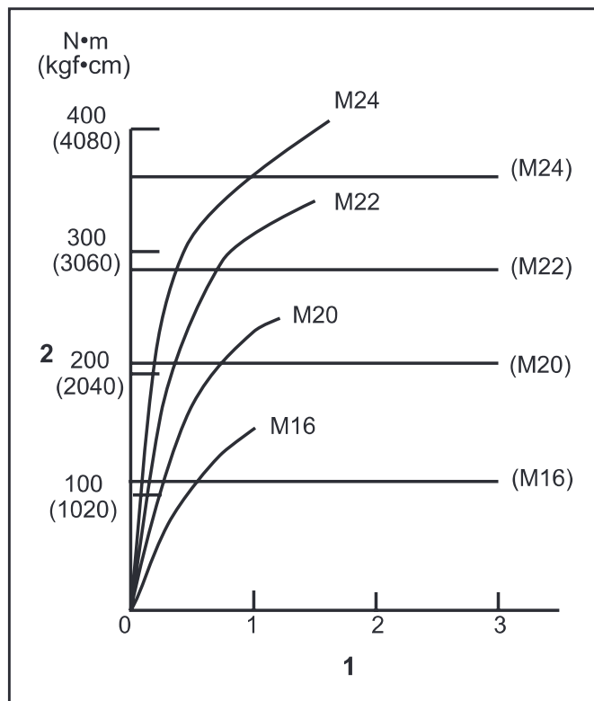
1. Pievilkšanas laiks (sekundēs) 2. Pievilkšanas griezes moments
