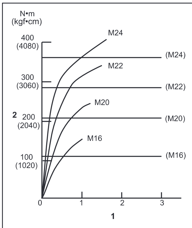
1. Užveržimo laikas (sekundėmis) 2. Užveržimo sukimo momentas
