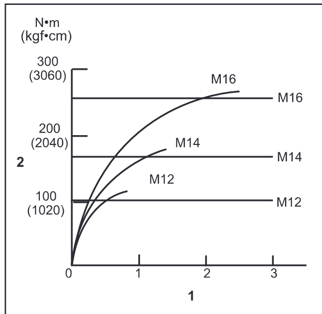
1. Tilspændingstid (sekunder) 2. Tilspændingsmoment
