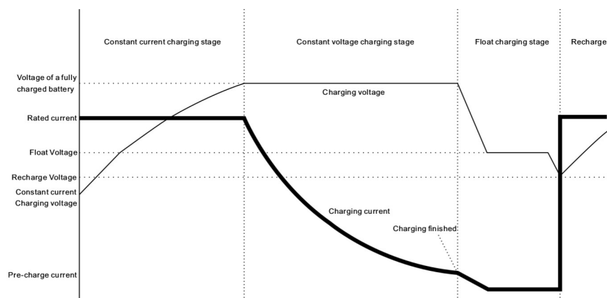
OPLADNINGSFASEDIAGRAM
