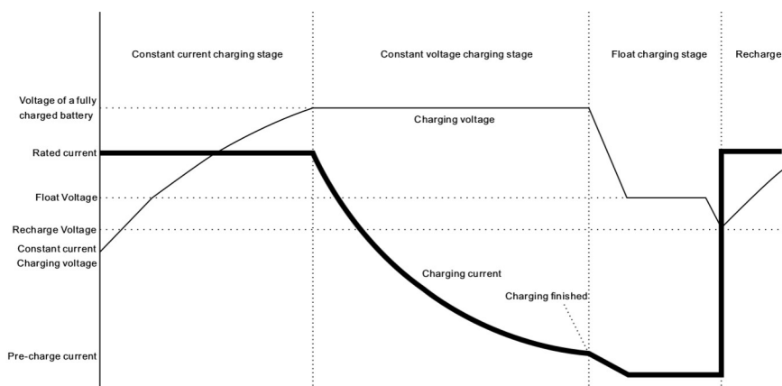
LADDNINGSTEGSDIAGRAM
