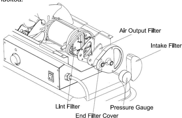
Kuva 6. Suodattimen vaihto
