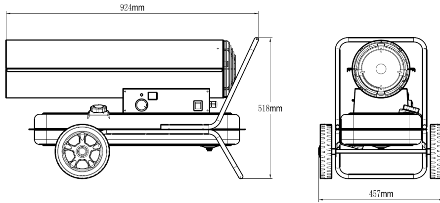
Kuva 2. Tuotteiden mitat
