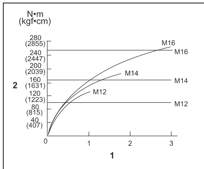
1. Åtdragningsmoment 2. Åtdragningsmoment
