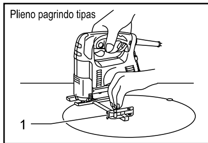
1. Kreiptuvas (kreipiamoji liniuotė)
