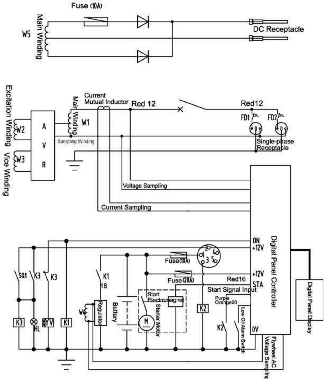
12.8 KDE6700TA Sähköinen kaavio (2)
