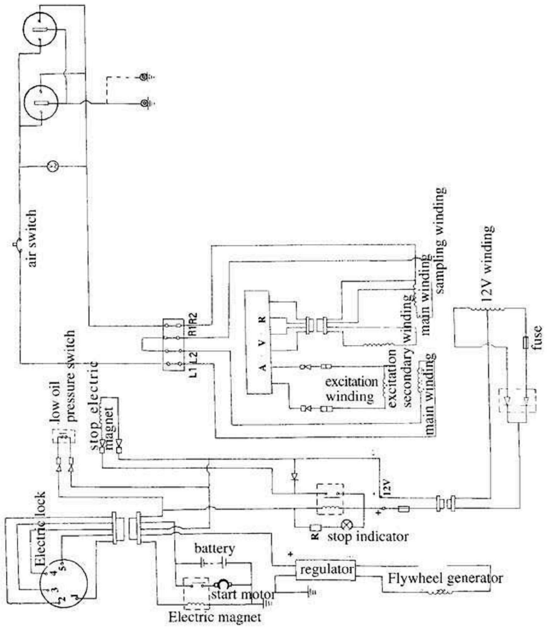
12.13 KDE2200E/KDE3500E/KDE5000E Sähköinen kaavio (yhellä jänniteulostulolla)
