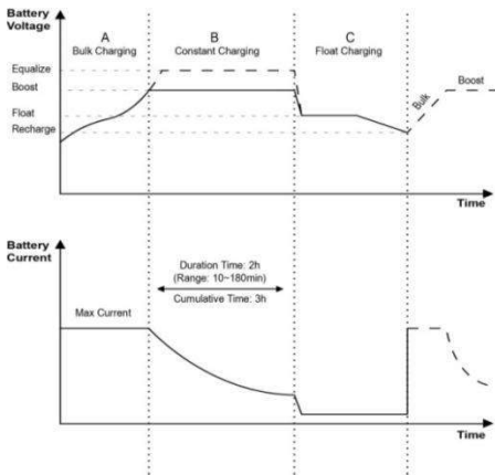
Kuva 1-4 Akun latauskäyrä
