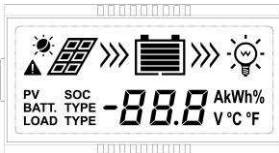
Kuva 3-1 LCD-näyttö
