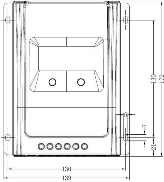
Tracer 2210A Mitat [mm]
