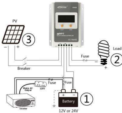
Kuva 2-1 Asennus
