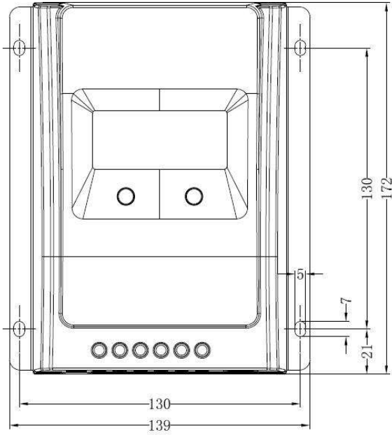
Tracer 3210A Mitat [mm]
