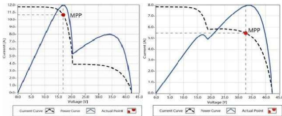
Kuva 1-3 Multi-MPP -käyrä
