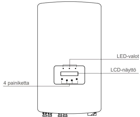
Kuva 1.1 Näkymä edestä
