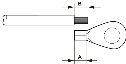
Kuva 5.8 Sopiva pituus
