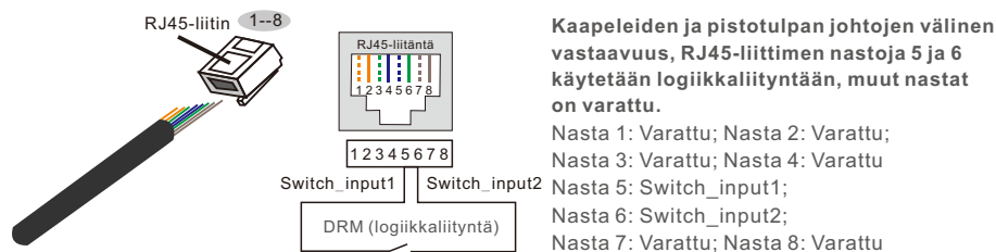
Kuva 5.31 Kuori eristekerrosta ja liitä RJ45-liitimeen.
