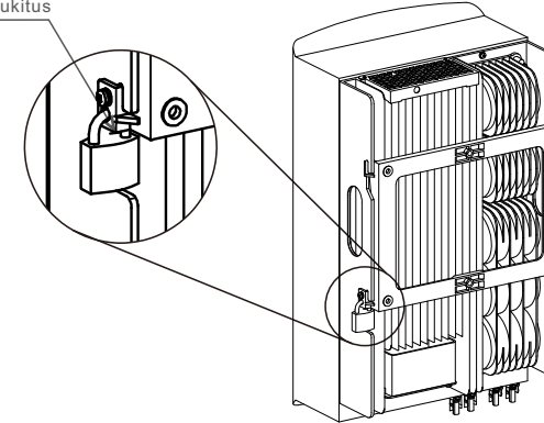
Kuva 5.7 Turvalukon asennus
