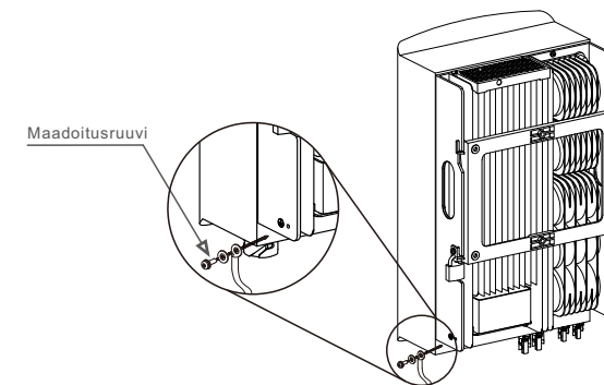
Kuva 5.10 Kiinnitetty kaapeli
