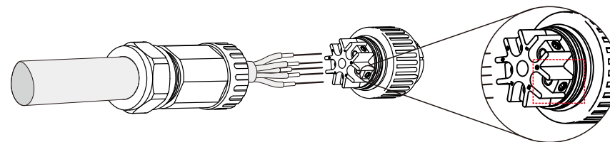
Kuva 5.22 Liitetty kaapeli
