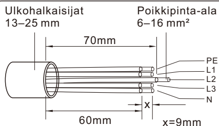
Kuva 5.20 Kuorittu ja paljas johto
