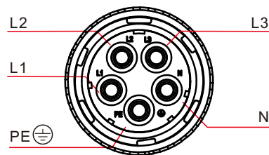
Kuva 5.21 AC-liittimen sisärakenne
