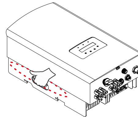
Kuva 4.2 Invertterin kahvat
