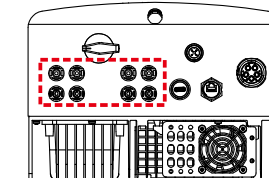
Kuva 5.18 DC-liittimien kytkeminen invertteriin
