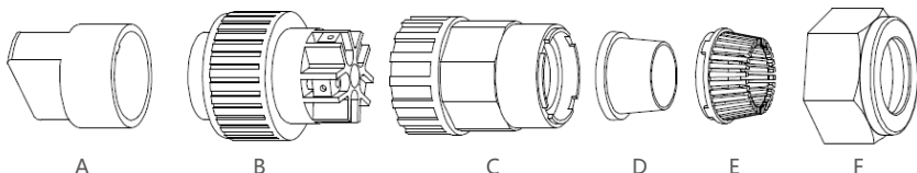
Kuva 5.19 AC-liitin
