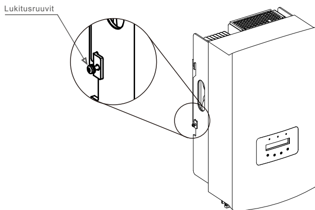
Kuva 5.6 Kiinnitä invertteri
