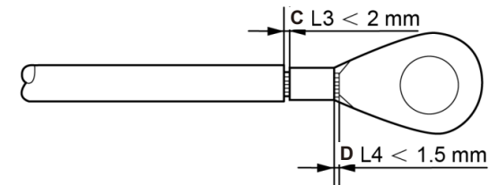
Kuva 5.9 Kuorittu johto
