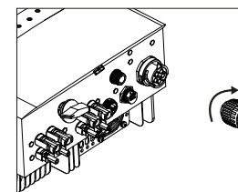
Kuva 5.24 AC-liittimen kytkeminen invertteriin
