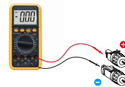
Kuva 5.17 Yleismittarin mittaus
