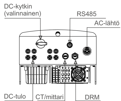
Kuva 1.2 Näkymä alhaalta
